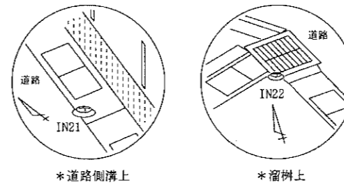
*引照点詳細図*
